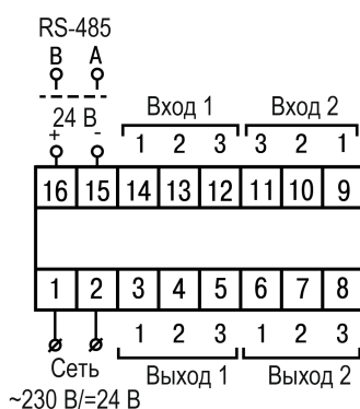
Рисунок 5.5 – Общая схема подключения 2TRM1–Ц5
