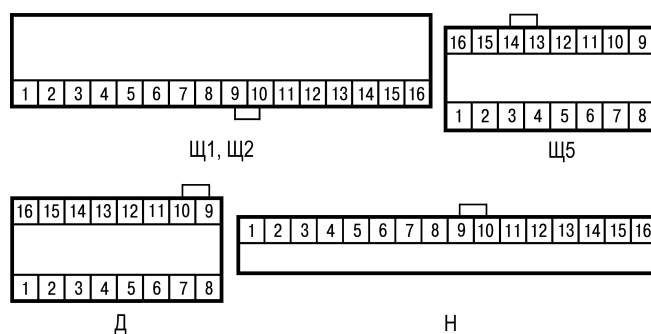
Рисунок 7.7 – Установка перемычки
