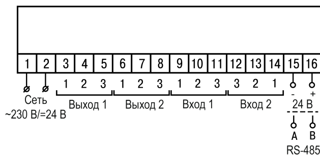
Рисунок 5.4 – Общая схема подключения 2ТРМ1–Щ1/Щ2
